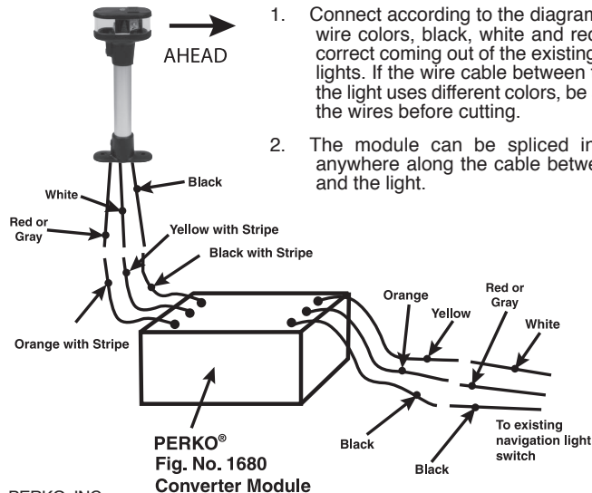
Fig. 1680 Wiring Diagram
